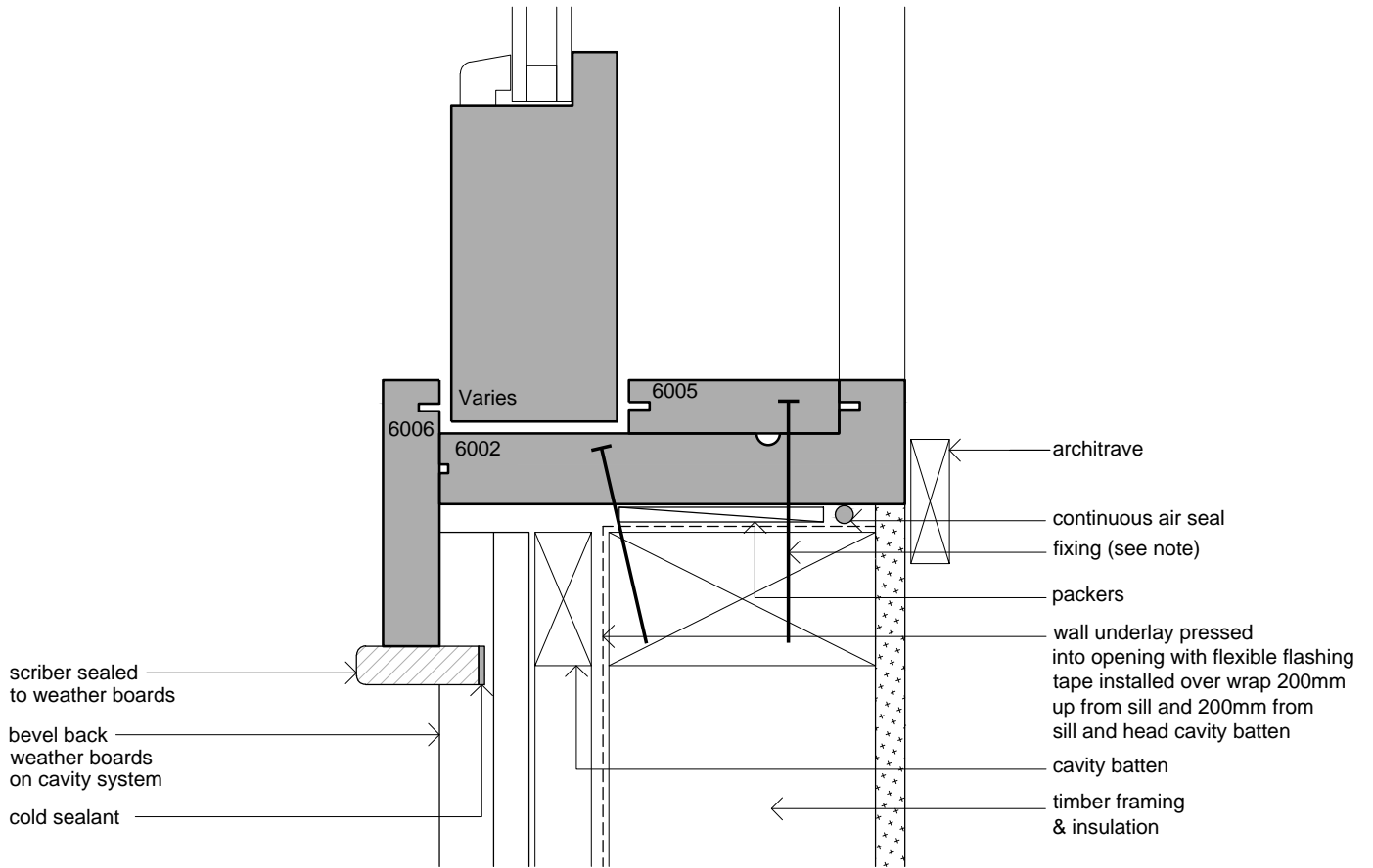
Window Jamb Scale: 1:2.5
