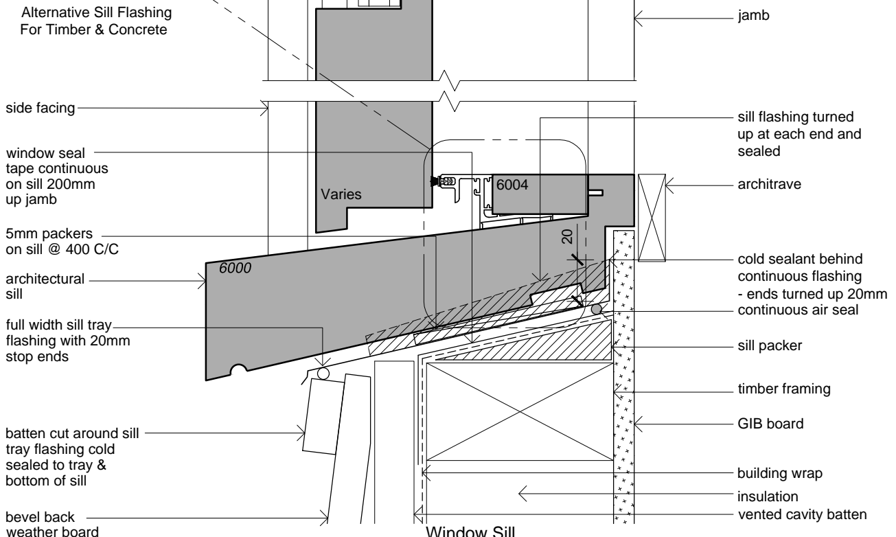
Window Sill Scale: 1:2.5
